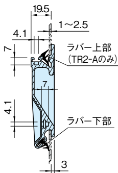
TR2-A (上部ラバー止め)
