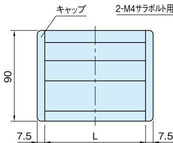
TR2-A (上部ラバー止め)
