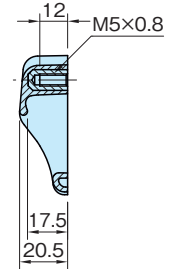
断面 X-X
