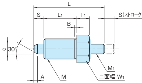
NDX-N NDX-N-SUS NDX-AN-SUS (シングルナット)
