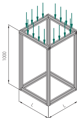
等分布荷重
