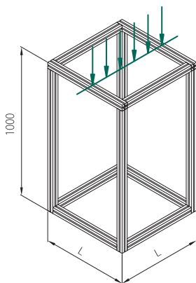
集中荷重
