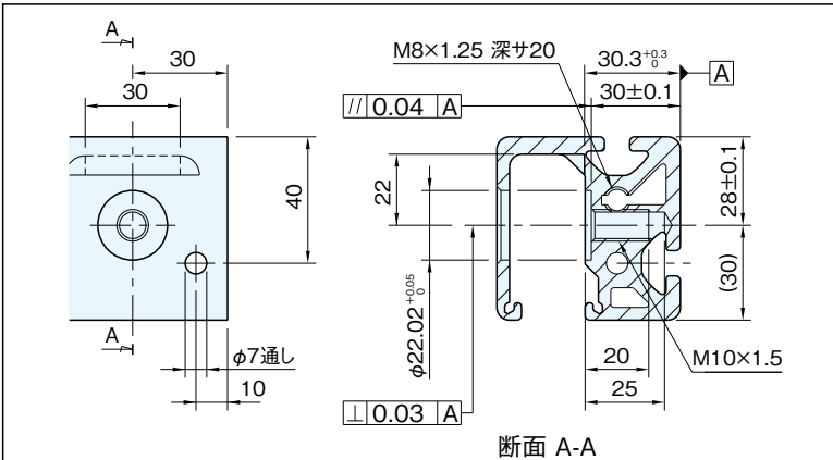
断面 A-A
