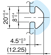
詳細 A
