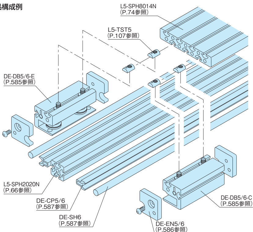
詳細図。
