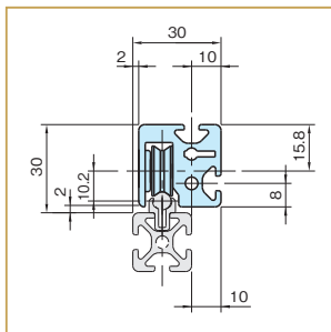
詳細図。
