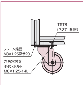
取付例。
