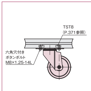
取付例。
