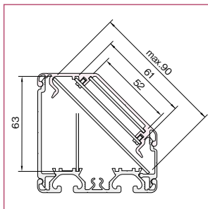
最大90mm幅までの基板が固定できます。
