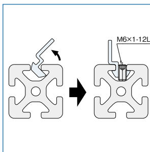
取付方法。
