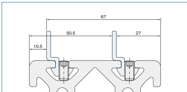
取付寸法。
