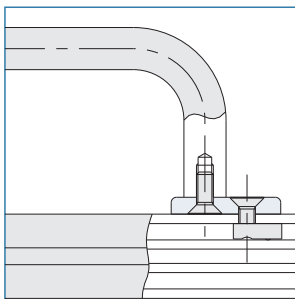
プロファイル取付方法。
