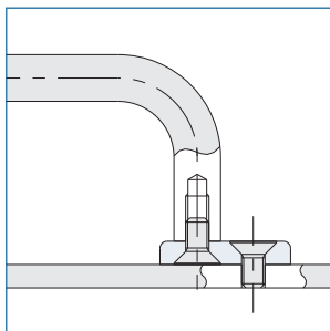
パネル取付方法。
