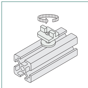
樹脂部が回転しますので、引き戸や折りたたみ ドアにご使用できます。
