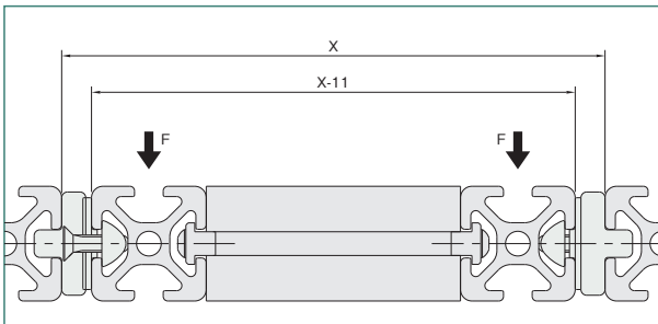
ナット グライダーはプロファイル溝にナットで 折りたたみドアの取付。(4ヶ使用) 固定してください。
