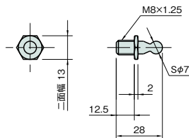
キャッチ用ボルト
