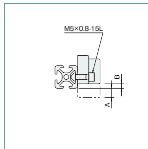
L5-SPH2020NIに取付けた場合の取付位置 A=9mm、B=4mm。
