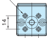
エンドプレート詳細 (両端面)
