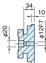
断面 A-A (3箇所)
