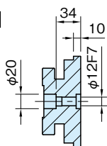
断面 A-A (2箇所)
