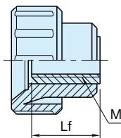
FTK-T (メネジ貫通)
