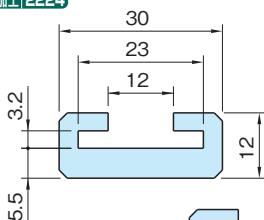
取付図
