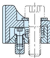
断面 X-X
