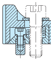
断面 X-X
