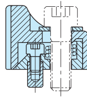
断面 X-X
