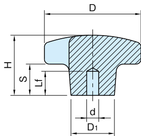
CK-C (下穴)
