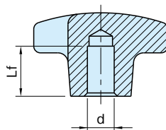
CK-R (精度穴)
