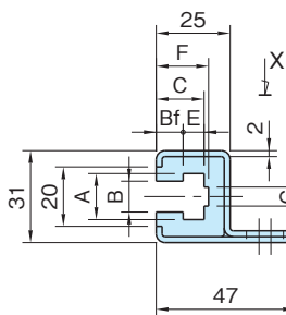
CGOC-B (Bタイプ)
