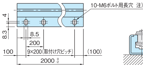
矢視 X
