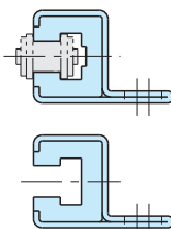
CGOC60Bの溝形状
