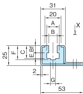
CGOC-A (Aタイプ)
