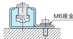
注) 取付けにはM6座金を使用ください。
