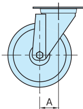
CAF8-SBL CAF8-SBL-SUS (旋回,プレート)
