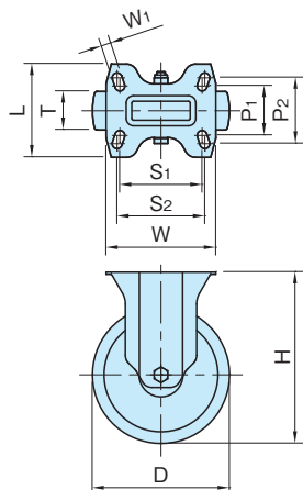
CAF8-PBL CAF8-PBL-SUS (固定)
