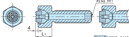
BUH-F 10015~24100 (フラットタイプ) BUH-E 10015~24100 (樹脂タイプ)
