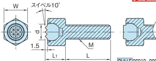
BUH-S 06012~08040 (セレーションタイプ)
