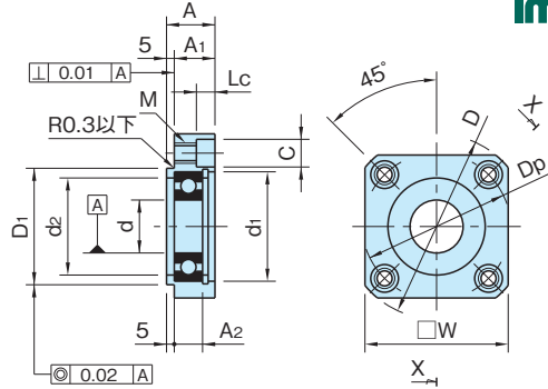
断面 X-X
