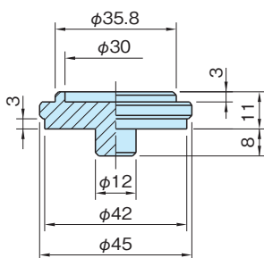
BJ733-12080 (ジョイントチップ)
