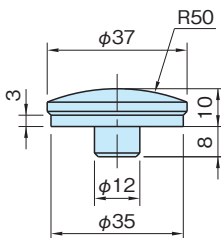
BJ733-12100 (球面チップ)
