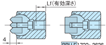
BBU-F 1722~3636 (フラットタイプ)
