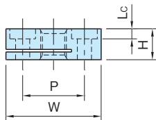
AMBV (垂直固定タイプ)
