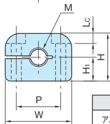
AMBH (水平固定タイプ)
