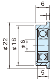
GRL2206P-L-SUS
