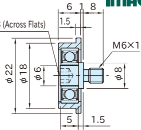
GRL22M6P-L-SUS
