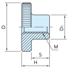
TKN TKN-SUS (内螺纹贯通孔)
