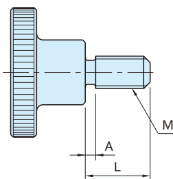
TKS TKS-SUS (外螺纹)
