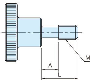
TKS-R-SUS (外螺纹、防止脱落型)
