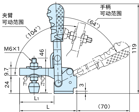
ST-VTC202U ST-VTC202U-S
