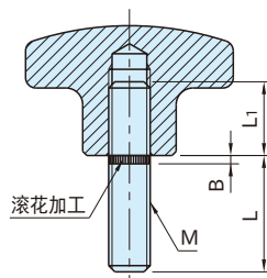
CK-SUS (外螺纹)
