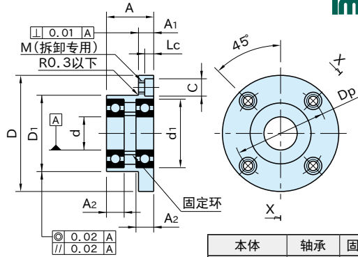
剖面 X-X
