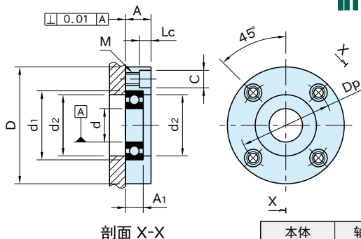
剖面 X-X
