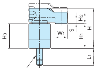
M1 内六角螺栓
