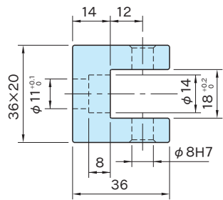
AR-3 (叉子)
