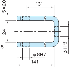
AR-2 (张力靴)
