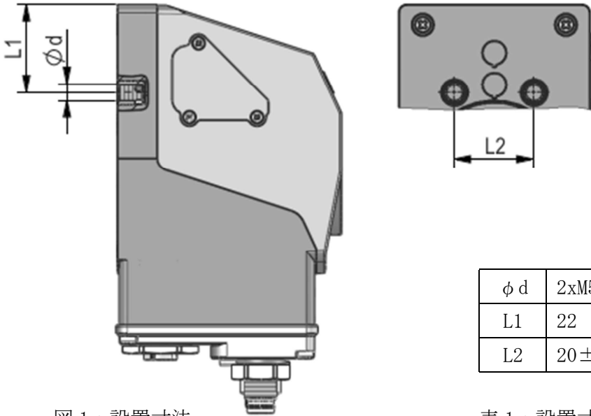
図 1：設置寸法
