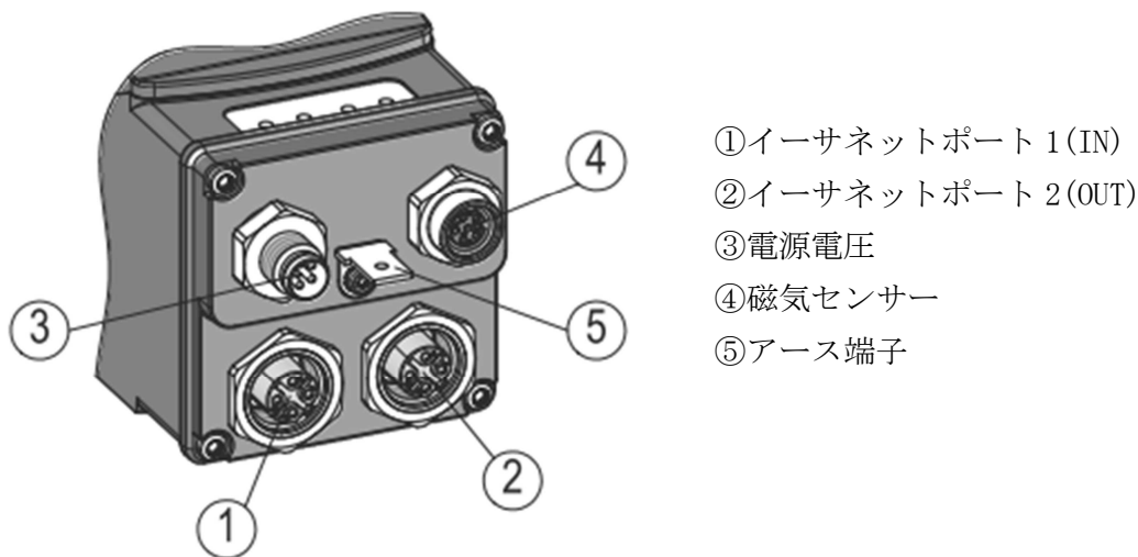
図2：コネクタ配置
