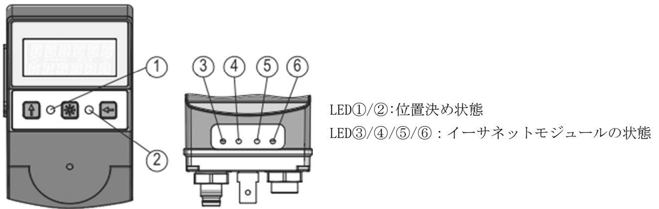
図 4 : LED 表示
