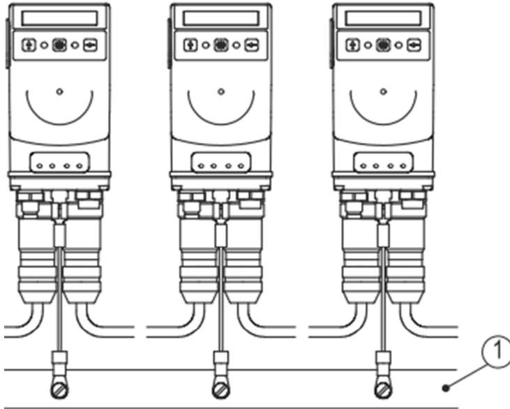
図 3 : アースバー
