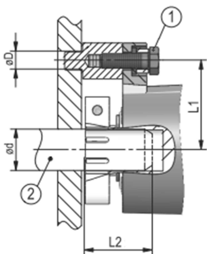
図1：設置寸法
