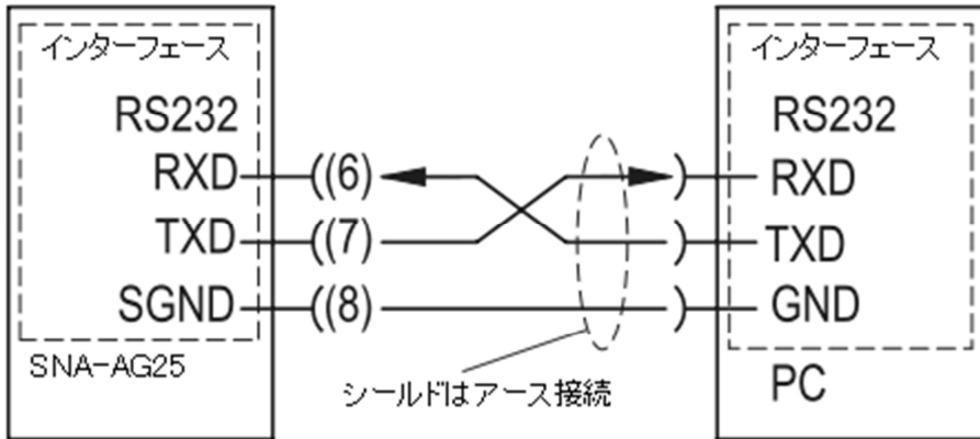
図 7 : RS232 インターフェースのピン配置
