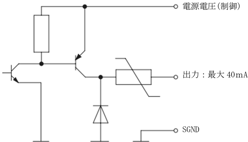
図 5 : 出力回路
