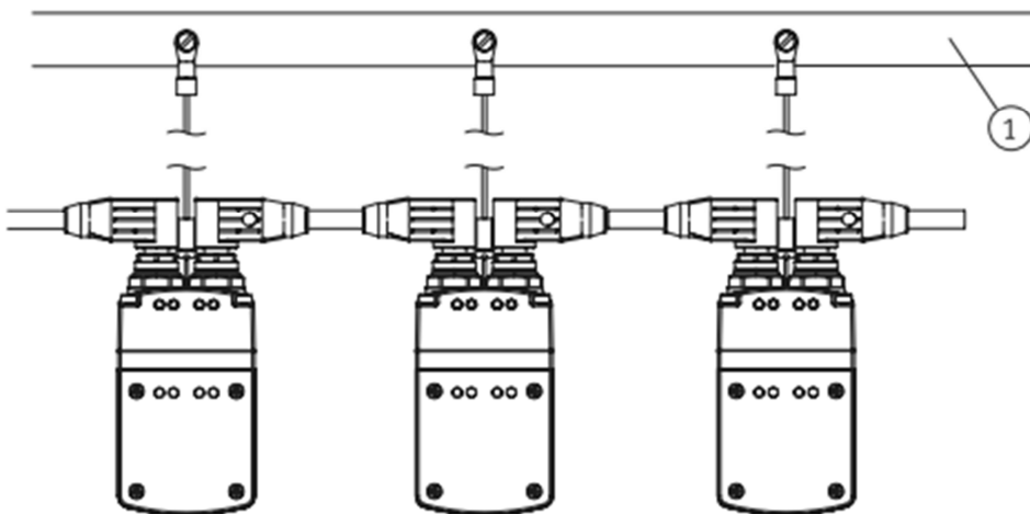
図 8 : アースバー
