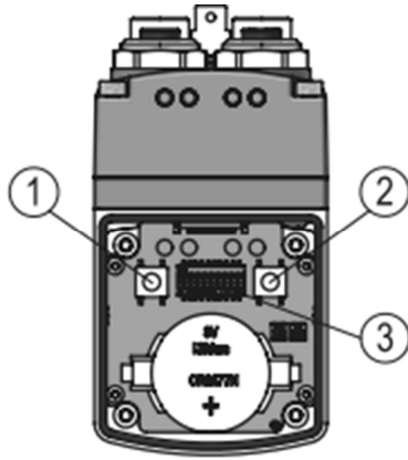
図 10：制御
