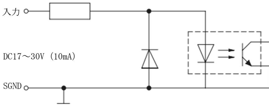
図 6 : 入力回路
