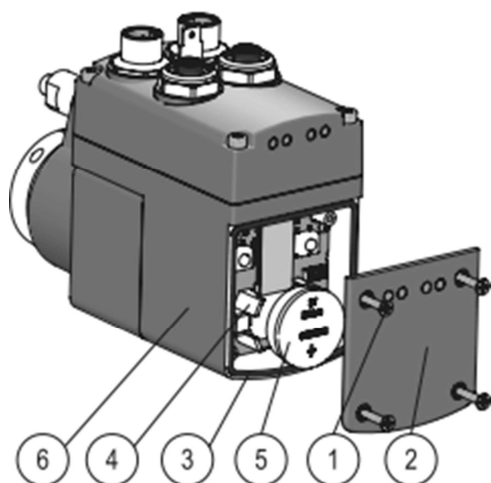
図 11 : バッテリー交換
