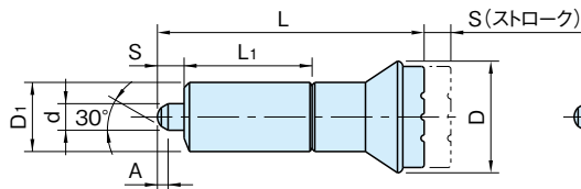
WDX WDX-SUS (ノーズロック無し)
