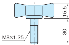
TMY830 (Oリングなし)
