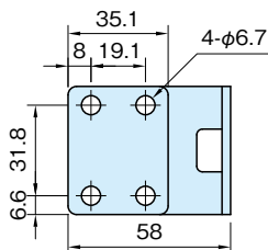
ST-PAH331 取付け詳細
