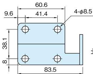
ST-PAH341 取付け詳細
