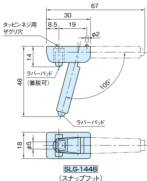
SLG-1448 (スナップフット)
