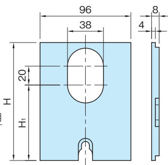
ワークサポートプレート (2個1組)
