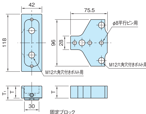
固定ブロック
