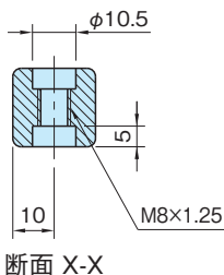
断面 X-X
