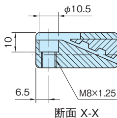
断面 X-X
