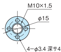
丸ナット
