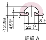
詳細 A
