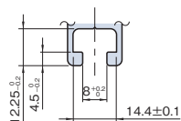
詳細 B
