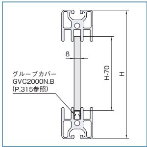
スライドドアパネル加工寸法。
