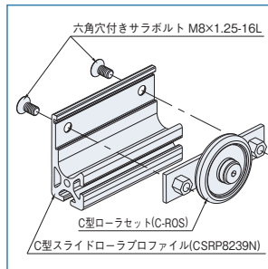
C型スライドローラユニットの部品構成。
