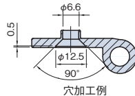
穴加工例
