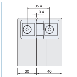
L6-HZN30-6/8の組み合わせパターン。
