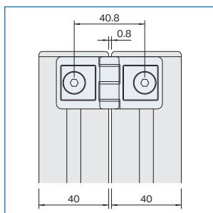
HZN30-8/8の組み合わせパターン。
