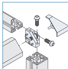
プロファイルへの加工はM8×1.25深サ20で加工してください。
