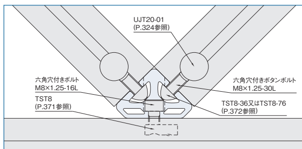
TナットSTはAJL4040Nの場合はTST8-36、AJL4080Nの場合はTST8-76で取付けてください。
