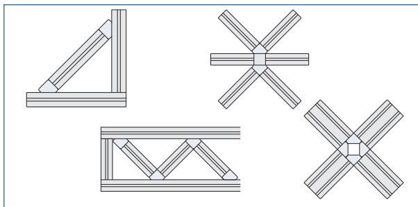
45°で2本のプロファイルの接続に。
